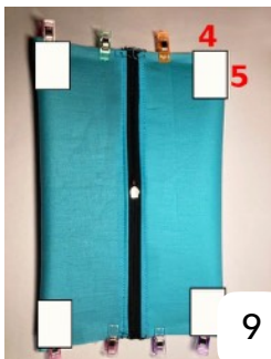
V rozích vystříháme dle fotky obdélníčky o velikosti 5 x 4 cm
